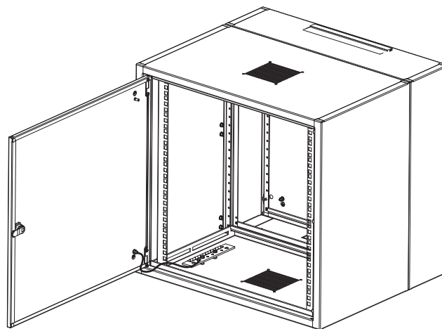
Заземление стальной двери в шкафу с шиной заземления
